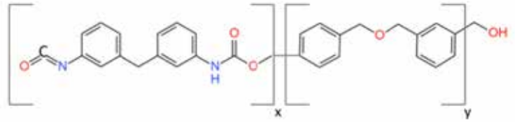
Şekil 2: Kutu Reçinesi Yapısı
